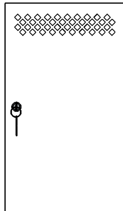
PERFORACJA W POSTACI ROMBU
